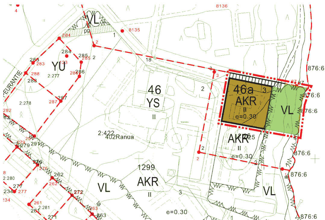
Kuva 9. Asemakaavaehdotus.
