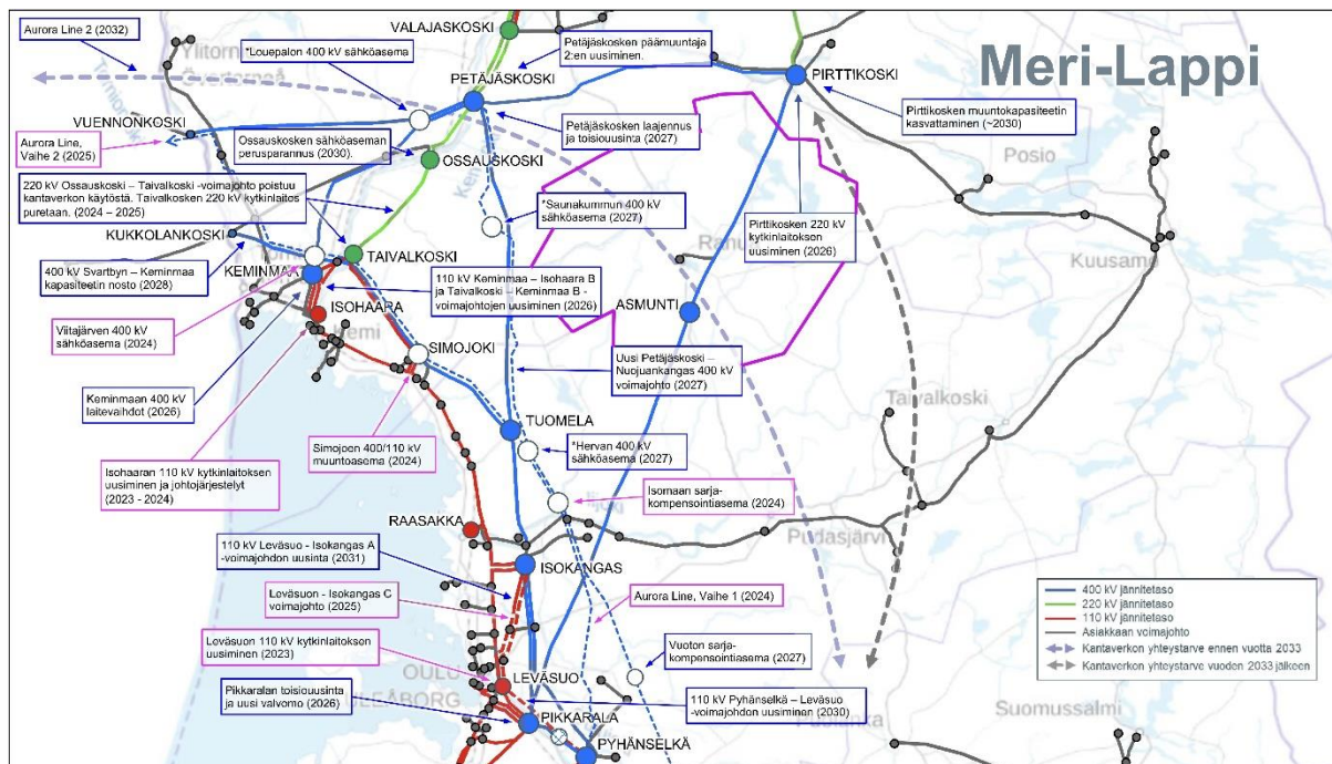
Kuva 23. Ote Fingridin kantaverkon kehittämissuunnitelmasta 2024–2033 (Fingrid). Ranuan kuntarajat lisätty karttaan violetilla rajauksella.
