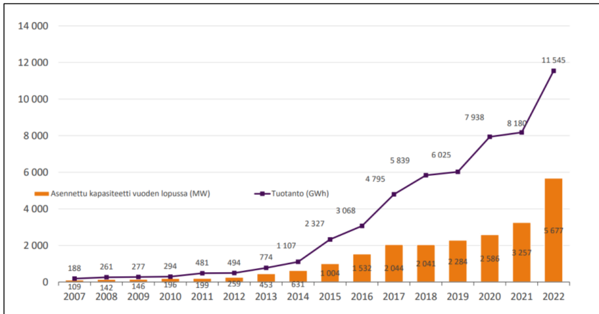
Kuva 4. Suomen tuulivoimatuotannon kehitys. Vuoden 2022 lopussa yhteiskapasiteetti oli 5677 MW (Energiatiedot 2023).
