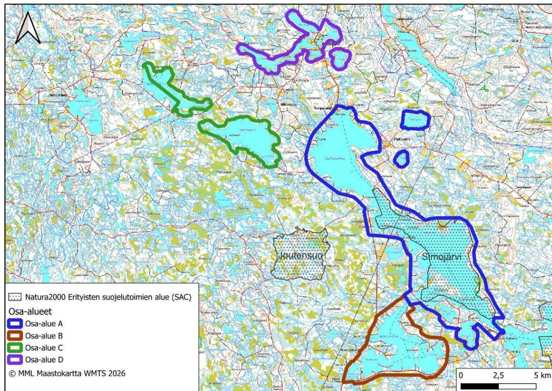
Kuva 26. Natura-alueet selvitysalueella
