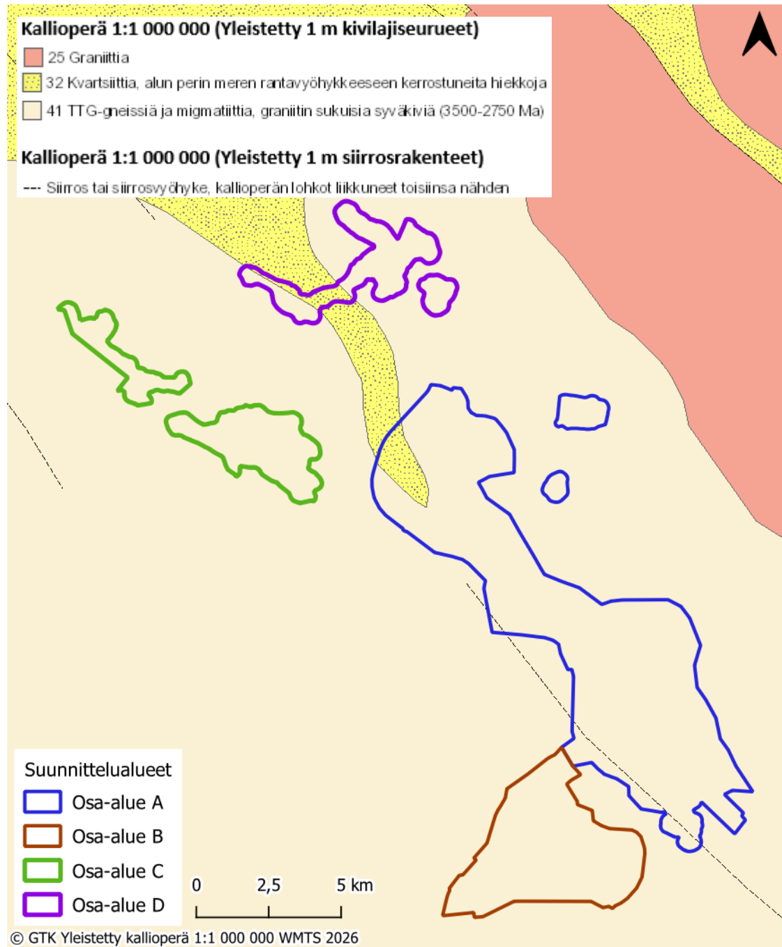
Kuva 18 Suunnittelualueen kallioperä.
