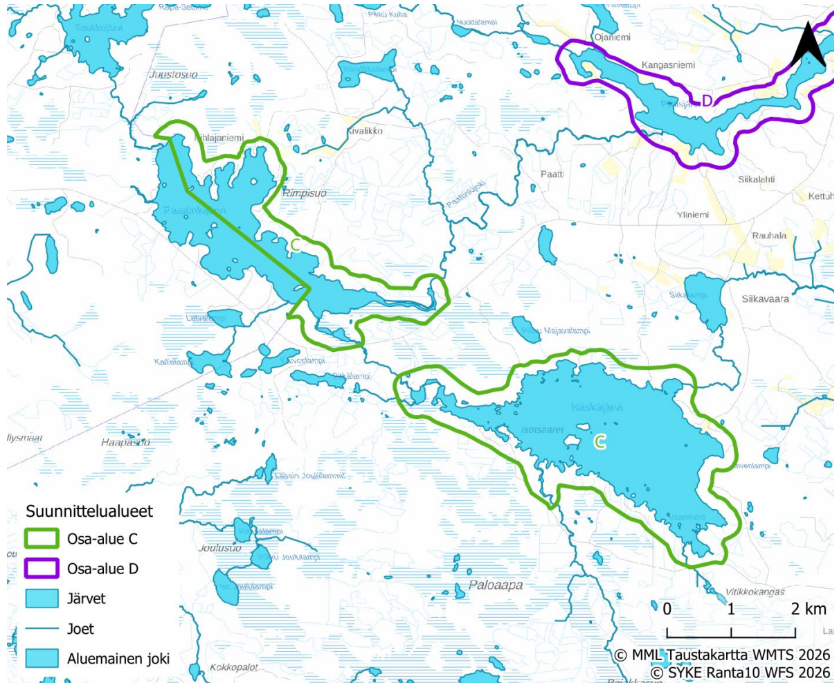
Kuva 19 Pintavesialueet suunnittelualueella.
