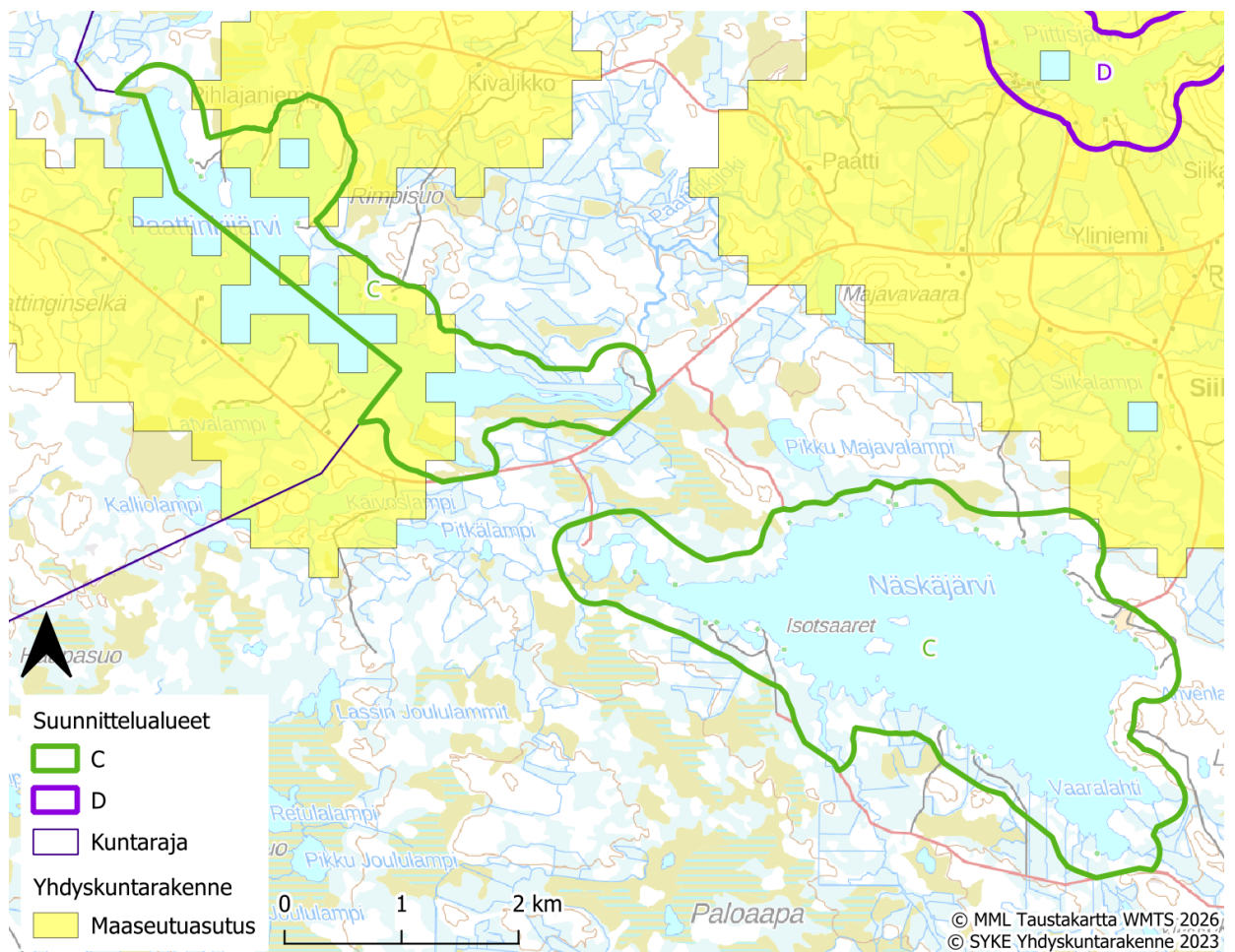
Kuva 5 Suunnittelualueen yhdyskuntarakenne
