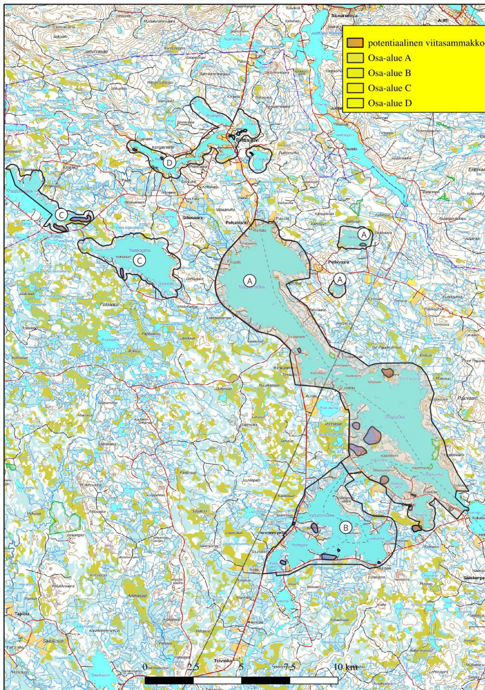
Kuva 37 Potentiaaliset viitasammakkoalueet.
